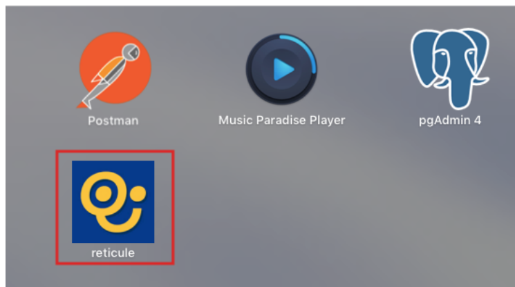
Изображение 4
