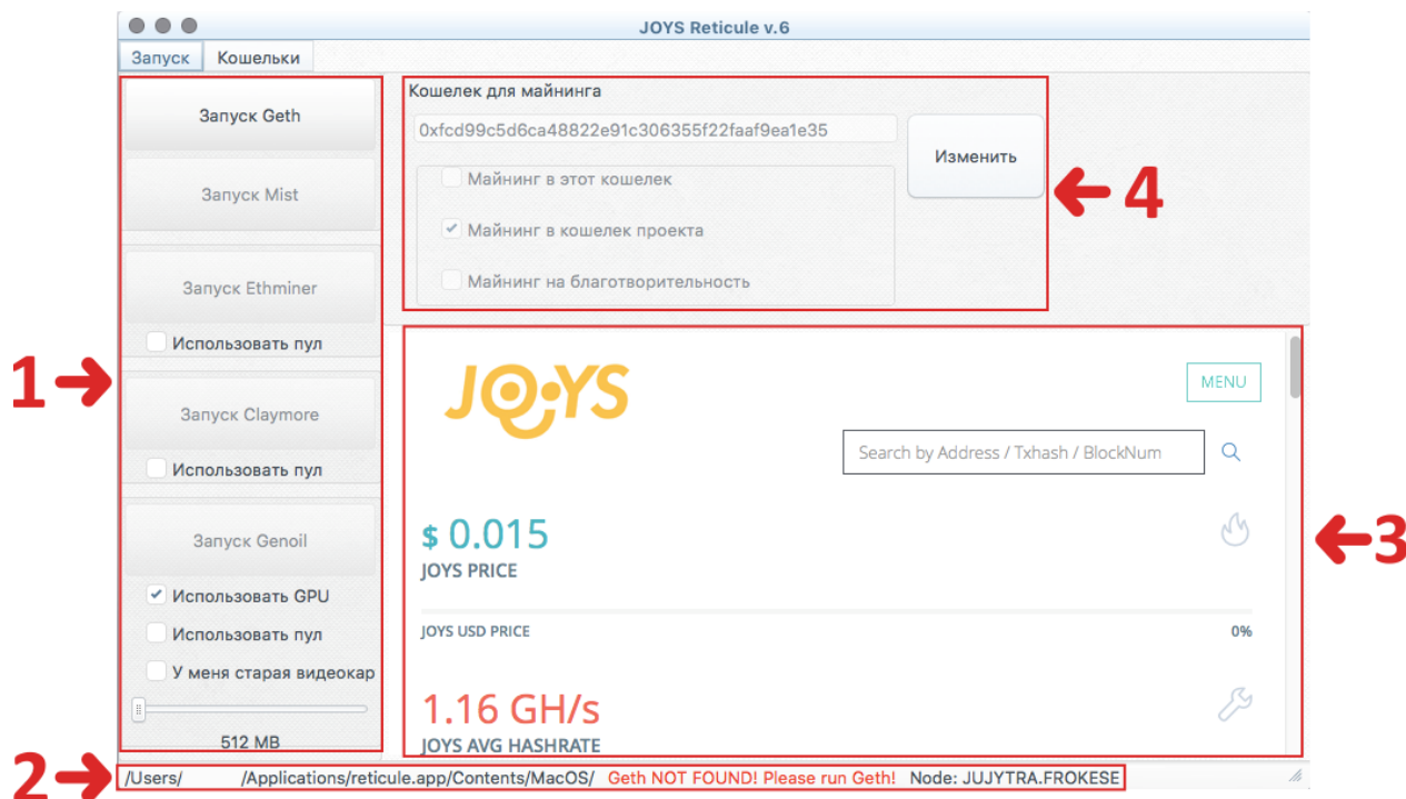
Изображение 5
